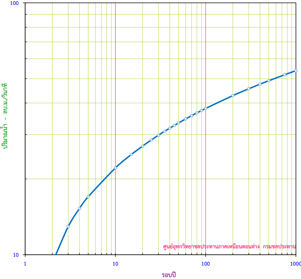
กราฟแสดง ปริมาณน้ำสูงสุดรายปี ขนาดรอบปีต่างๆ สถานี Y.29 อ.ศรีสัชนาลัย จ.สุโขทัย
